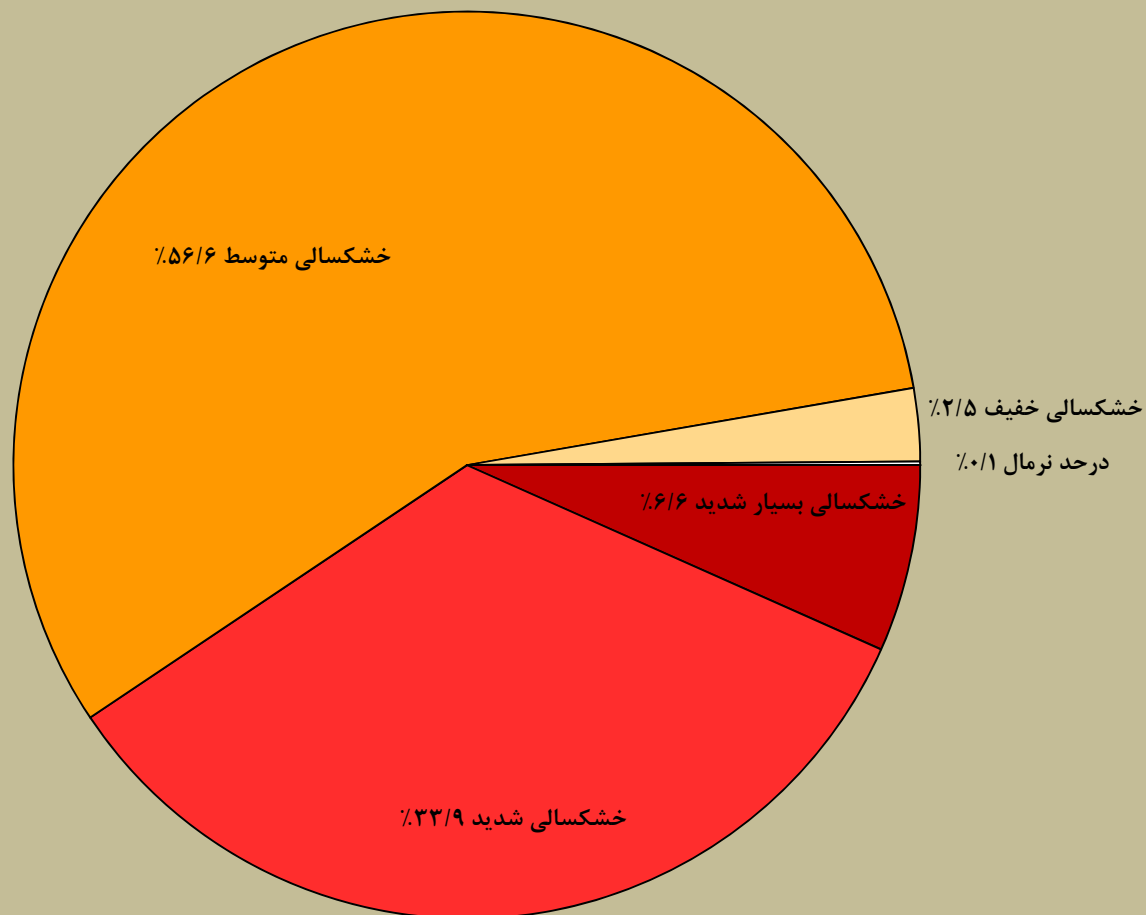
درصد مساحت تحت تاثیر خشکسالی براساس شاخص SPEI دوره هفت ساله تا پایان آذر ماه ۱۳۹۶ در سطح استان زنجان
